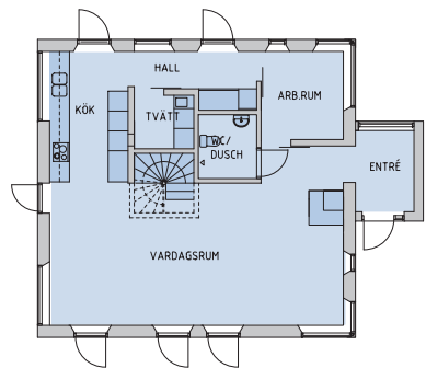
Plan bottenvåning
